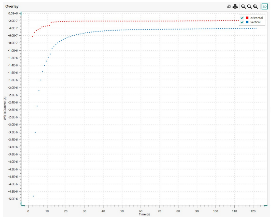
Testare amperometrica
